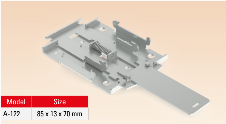
A-122 DIN RAIL MOUNTING KIT
