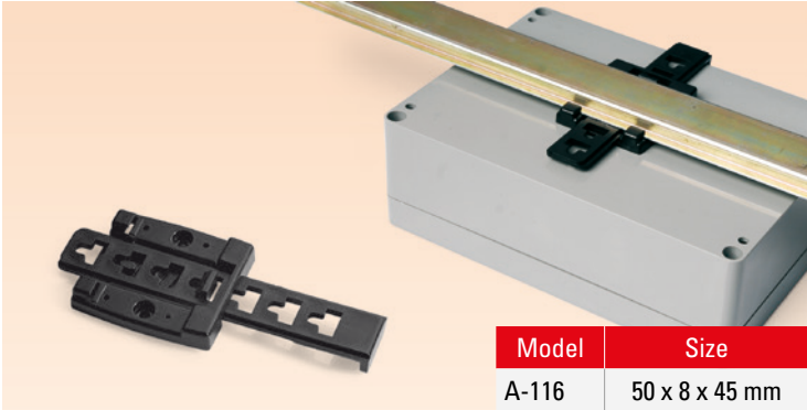
A-116 DIN RAIL MOUNTING KIT
