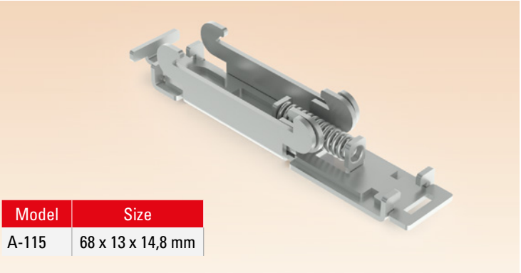
A-115 DIN RAIL MOUNTING KIT
